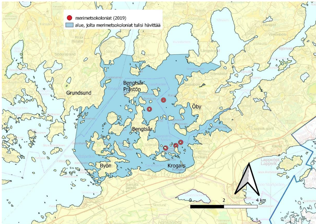
Kuva 14. Bengtsåran ympäristön merimetsokoloniatilanne vuonna 2019 sekä alue, jolta merimetsokoloniats tulisi kalatalousalueen näkemyksen mukaan suunnittelukauden aikana hävittää luonnonvaraisten kalakantojen turvaamiseksi. Aluerajauksessa on huomioitu mm. kaupallisten kalastajien ilmoittamat siian lisääntymisalueet ja Krogarsin EMMA-alue (Lappalainen ym. 2020). Sisältää Maanmittauslaitoksen aineistoa (2020).
