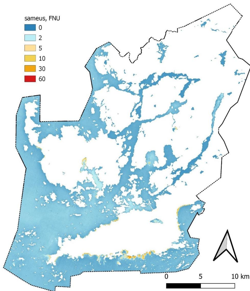
Kuva 4. Pintaveden sameuden keskiarvo vuosien 2015–2018 heinä-syykuun välisenä aikana. Kuva perustuu Suomen ympäristökeskuksen satelliittikuva-aineiston tulkintaan (Syke 2020). Sisältää Maanmittauslaitoksen aineistoa (2020).
